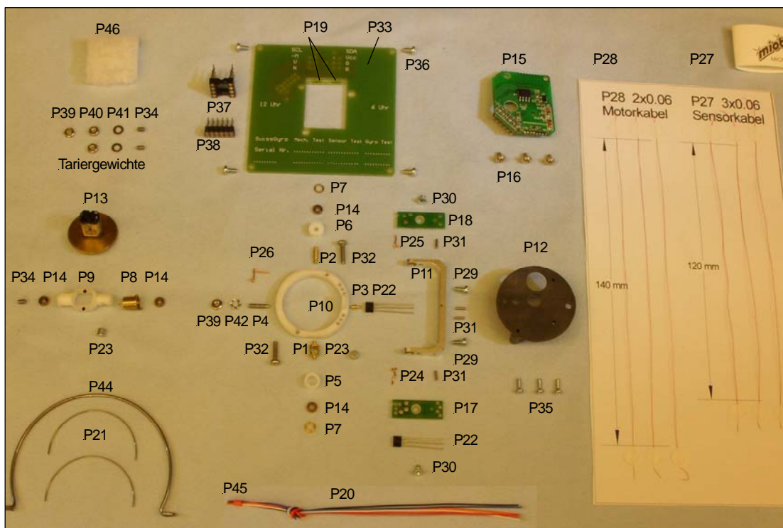
Fig. 2. Einzelteile des SwissGyro V2
