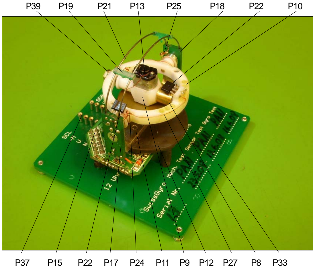
Fig. 1. Funktionsbereiter SwissGyro V2
